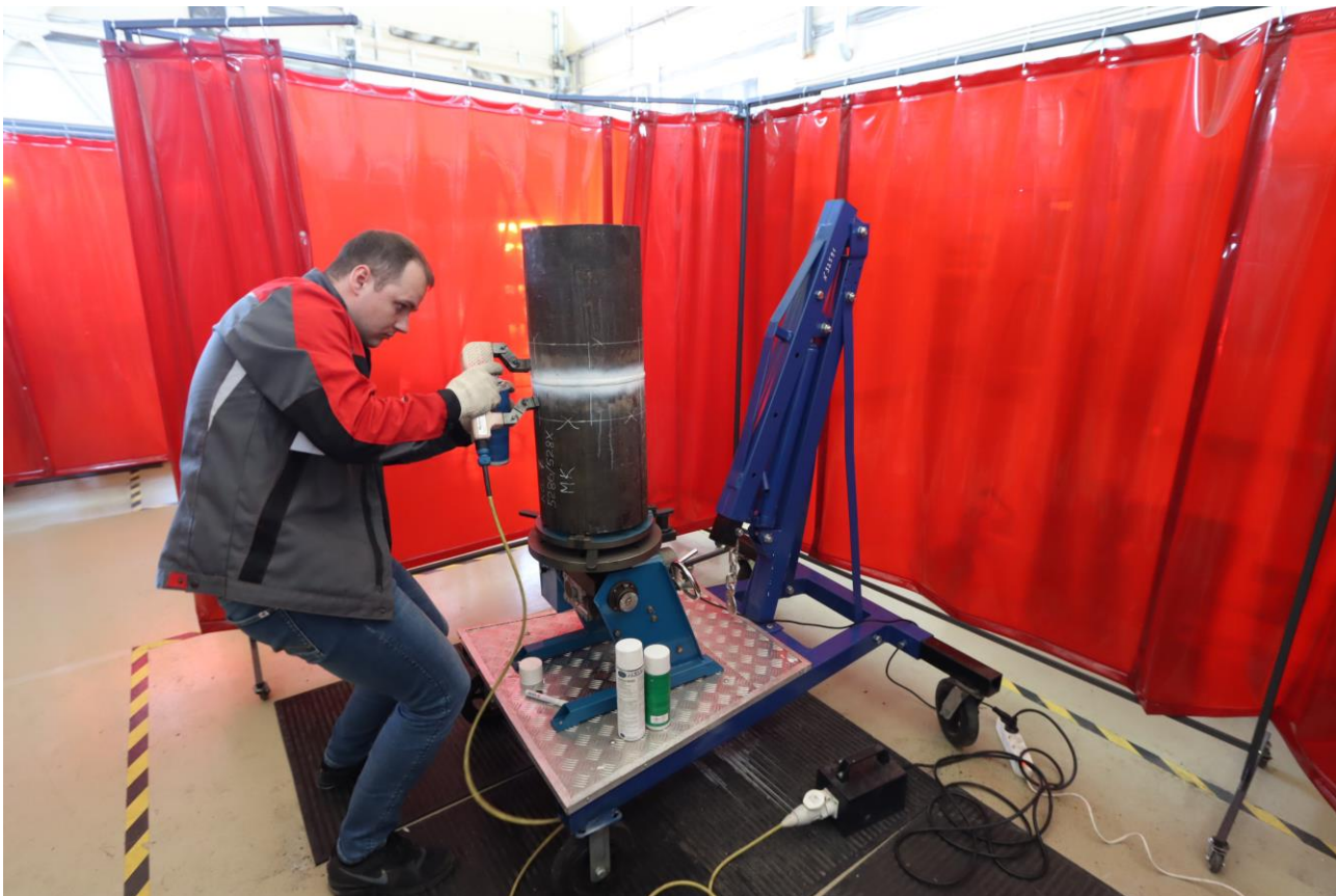
Участок для магнитопорошкового контроля качества КСС
