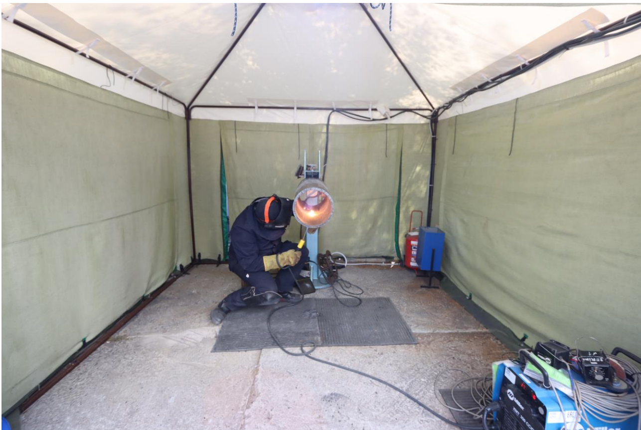
Сварочная палатка № 3 для ручной дуговой сварки КСС в положении Н45, ремонта сваркой
